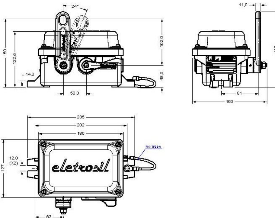
Chave de emergência DS-418 "simples" com montagem à esquerda
