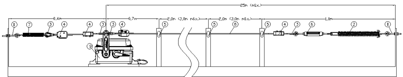
Chave de emergência DS-418 "simples" com montagem à direita
