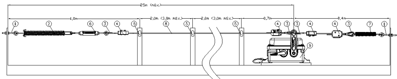
Chave de emergência DS-418 "simples" com montagem à esquerda
