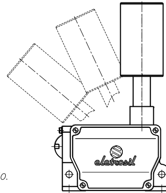
CHAVE COM MONTAGEM A ESQUERDA
